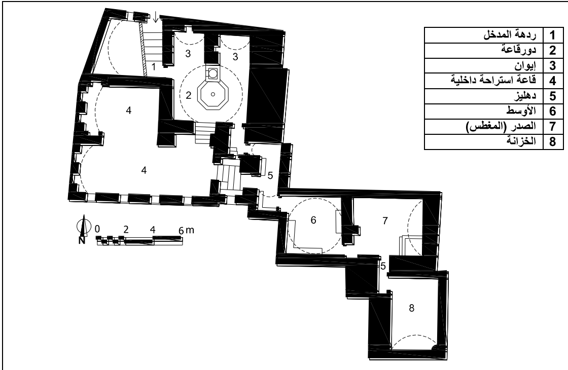
شكل (3) مخطط أفقي للحمام الكبير - عمل الباحث
